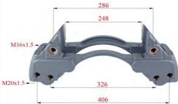
TK2211-02 KALİPER TAŞIYICI Caliper Carrier KNORR
